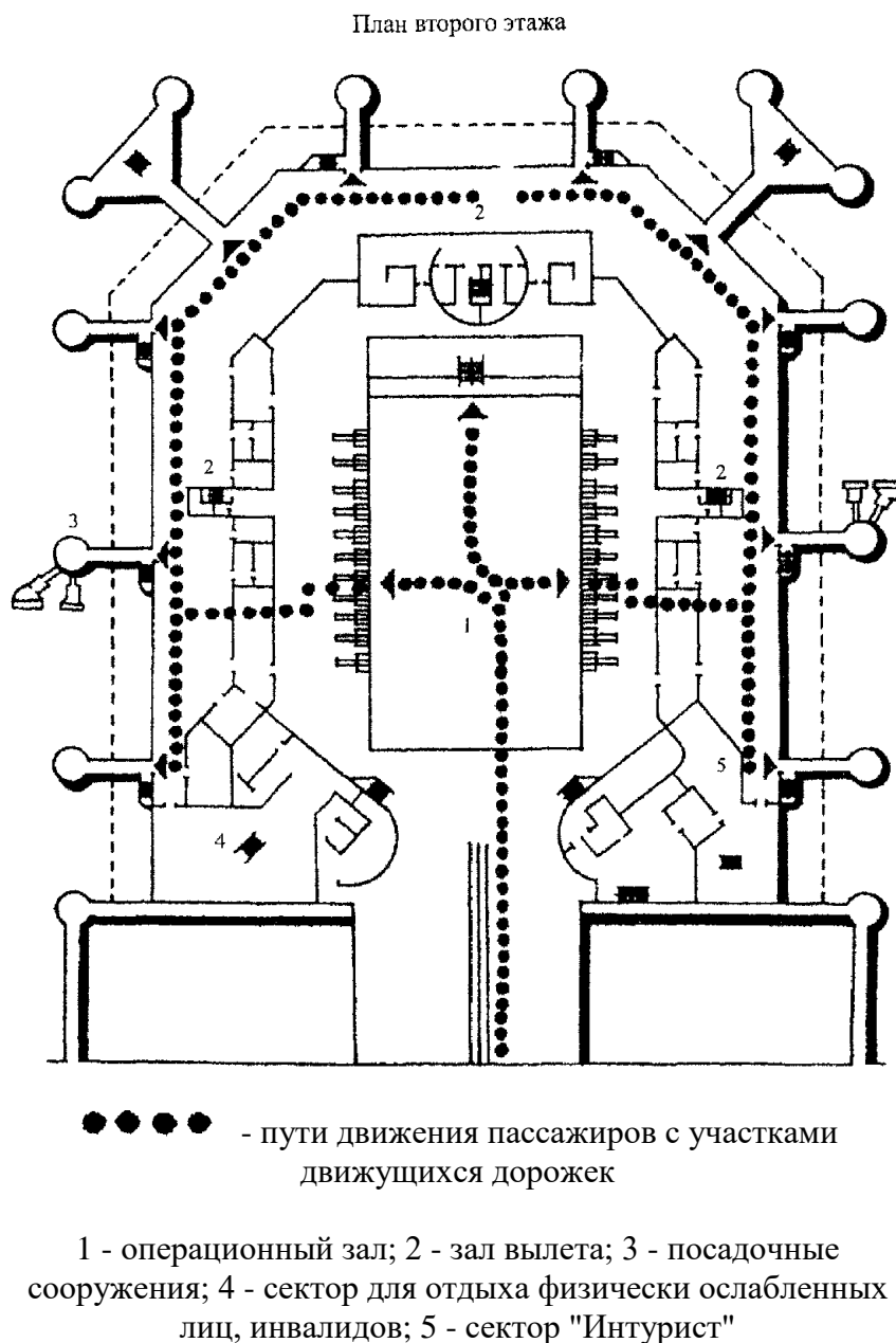
Рисунок В.13. Организация движения пассажиров в аэровокзале
